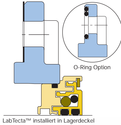
LabTecta™ installiert in Lagerdeckel
