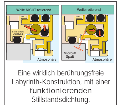
LabTecta™ integriertes Umgebungsfeuchtigkeits-Schutzsystem
