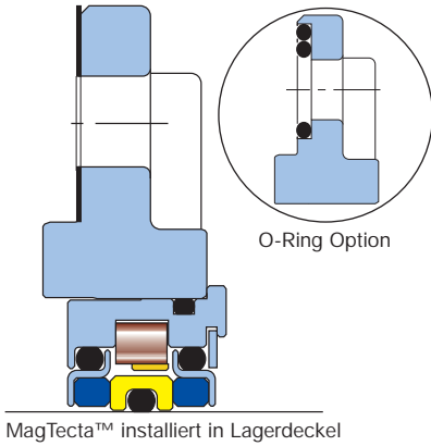
MagTecta™ installiert in Lagerdeckel
